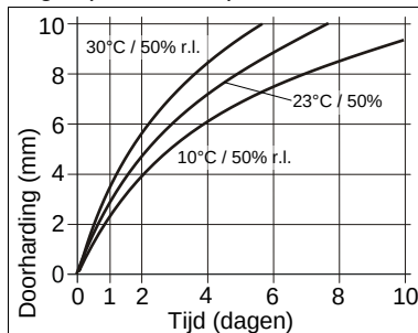
Schema 1: Doorhardingssnelheid voor Sika® Firesil Marine N
